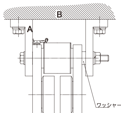
図-5 A、B共に磁性体の場合 非磁性体のワッシャーを片側に挟む
