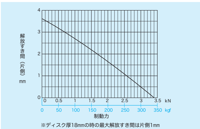
■NDB-400B型 解放すき間（片側）・制動力曲線（ \mu=0.33 ）
