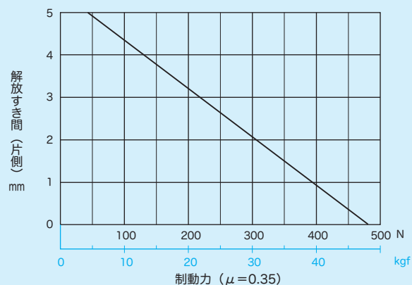
■NDB-20A型 初期解放すき間（片側）・制動力曲線 ( \mu=0.35 )
