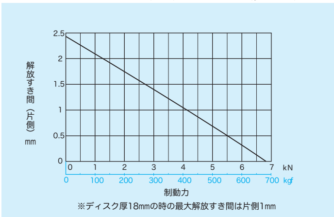
■NDB-1400A型 解放すき間（片側）・制動力曲線（ \mu=0.33 ）
