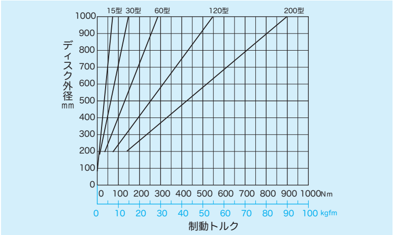
■ GDN型 ディスク外径・制動トルク曲線 ( \mu=0.33 )
