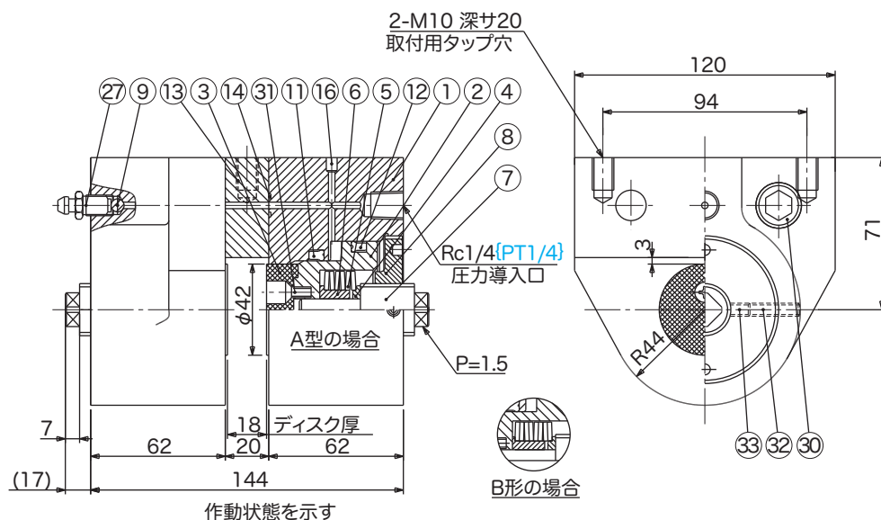
■ NDB-400型 部品表
