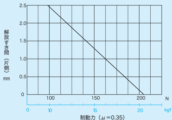
■NDB-10A型 初期解放すき間（片側）・制動力曲線 ( \mu=0.35 )
