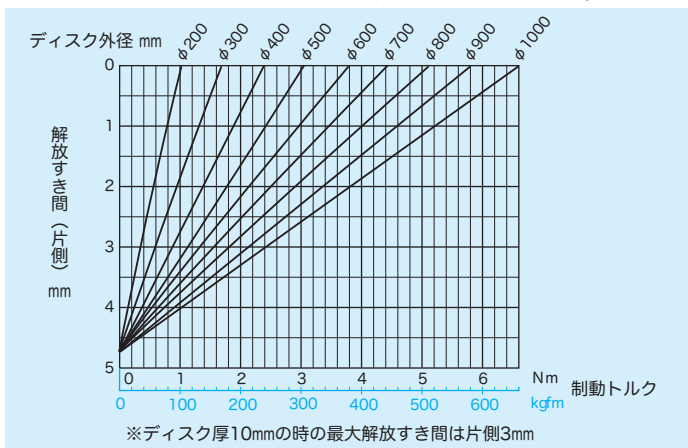
■NDB-1400B型 解放すき間（片側）・制動トルク曲線（ \mu=0.33 ）
