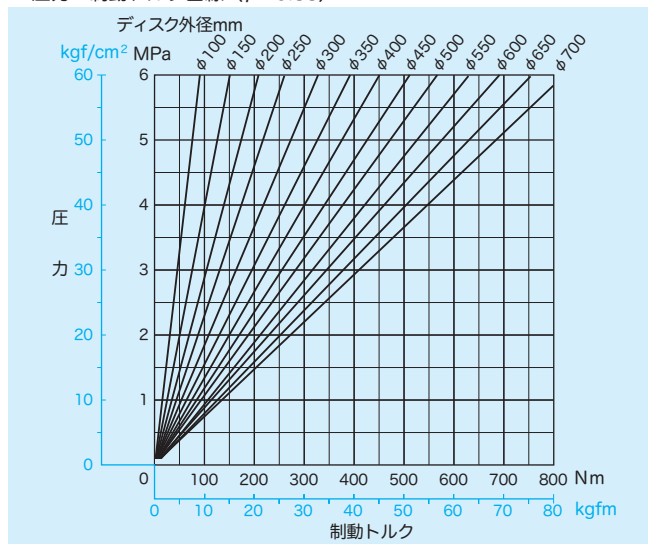
■DBL-20、RDB-20 圧力・制動トルク曲線 (μ=0.33)
