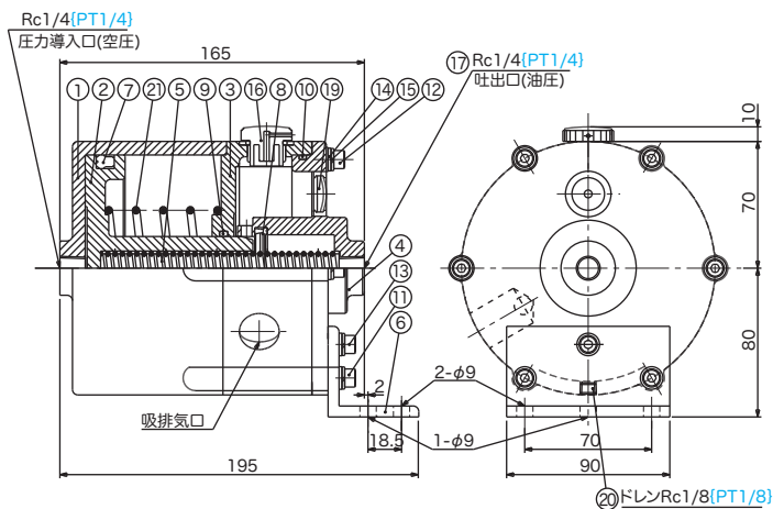
BO-20型 部品表
