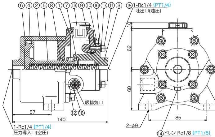
BO-10型 部品表
