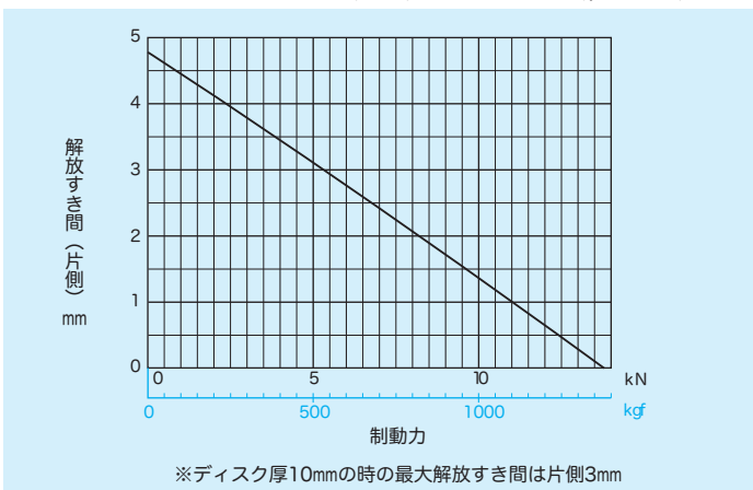
■NDB-1400B型 解放すき間（片側）・制動力曲線（ \mu=0.33 ）
