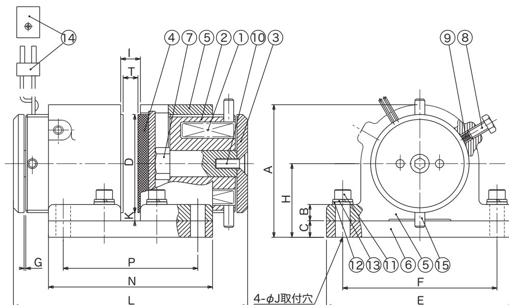
■ PGDB型 部品表
