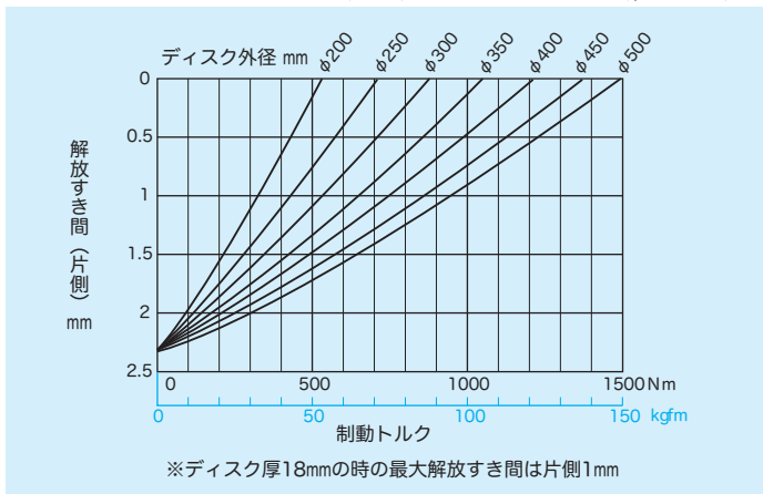
■NDB-1400A型 解放すき間（片側）・制動トルク曲線（ \mu=0.33 ）
