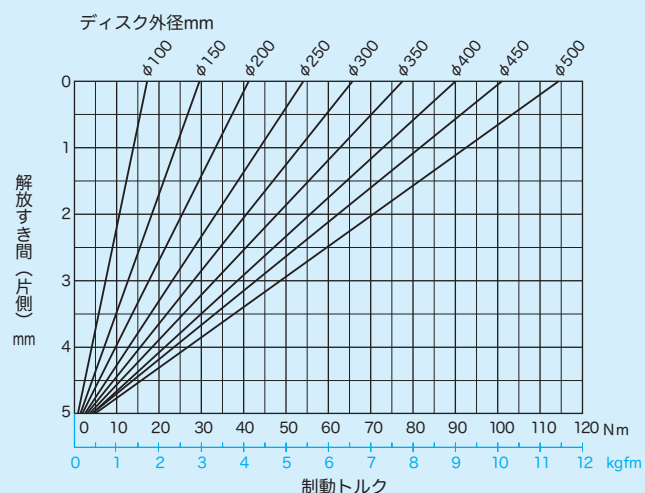
■NDB-20A型 初期解放すき間（片側）・制動トルク曲線 ( \mu=0.35 )
