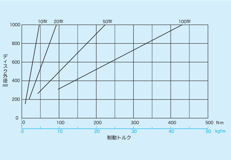
PGDB型 ディスク外径・制動トルク曲線 (μ=0.33)
