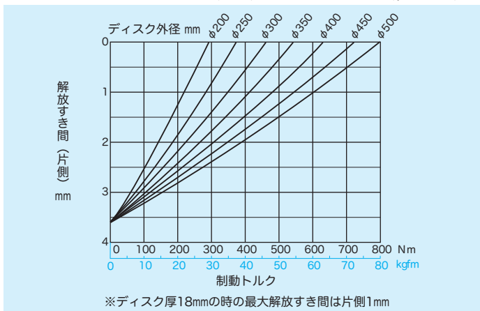
■NDB-400B型 解放すき間（片側）・制動トルク曲線（ \mu=0.33 ）
