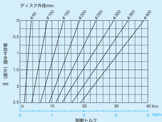
■NDB-10A型 初期解放すき間（片側）・制動トルク曲線 ( \mu=0.35 )
