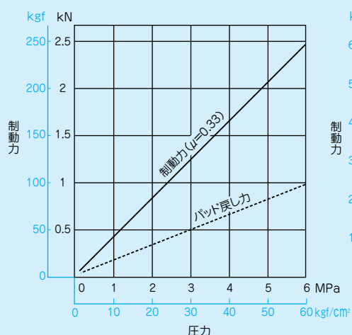
■RDB-10形
