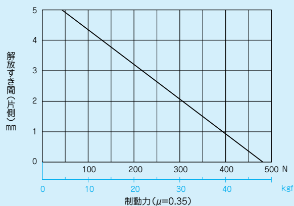
■NDB-20A形 初期解放すき間(片側)・制動力曲線( \mu=0.35 )
