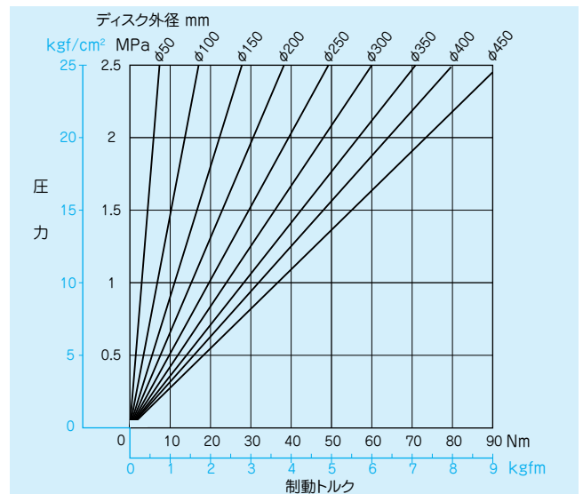
■ DBL-50、RDB-50 圧力・制動トルク曲線(μ=0.33)
