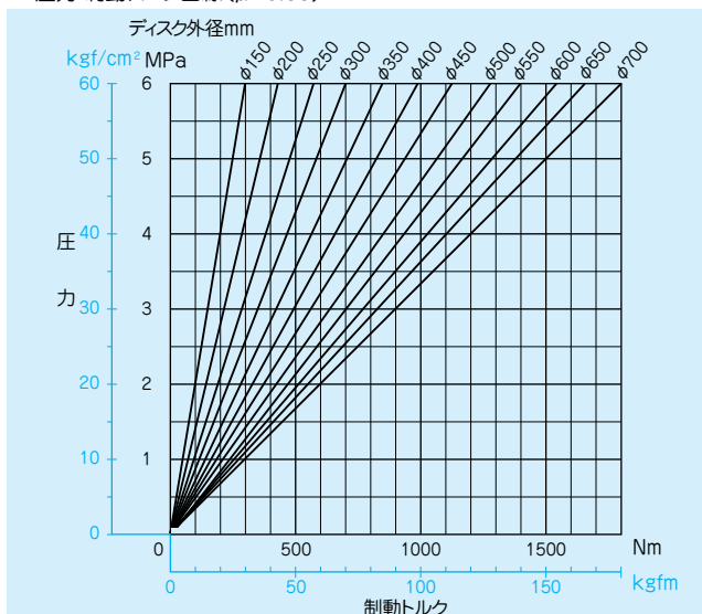
■DBL-20、RDB-20 圧力・制動トルク曲線 ( \mu=0.33 )
