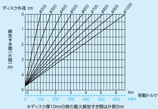
■NDB-1400B形 解放すき間(片側)・制動トルク曲線( \mu=0.33 )
