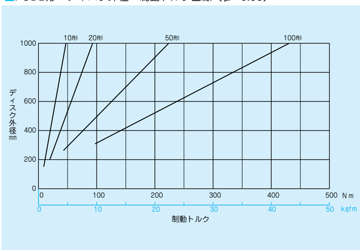
PGDB形 ディスク外径・制動トルク曲線 ( \mu=0.33 )
