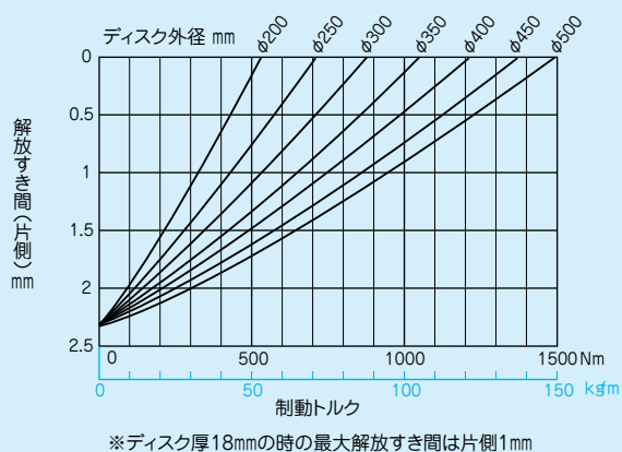
■NDB-1400A形 解放すき間(片側)・制動トルク曲線( \mu=0.33 )
