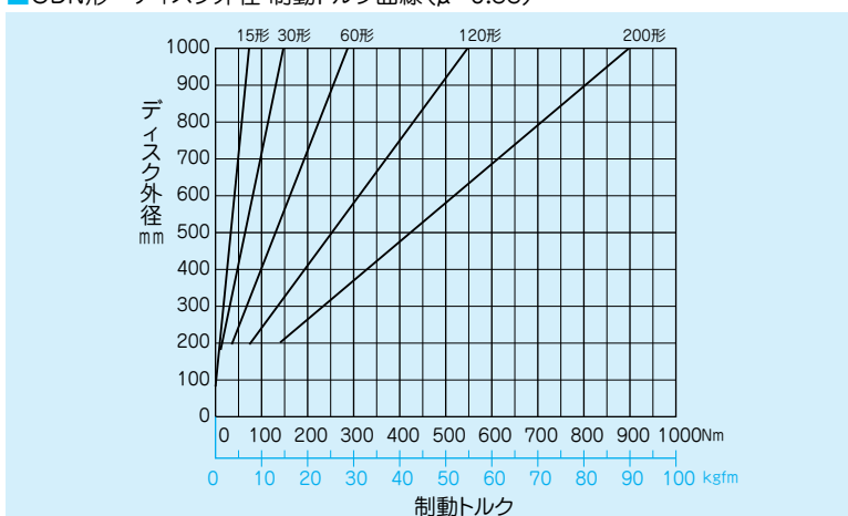
■GDN形 ディスク外径・制動トルク曲線( \mu=0.33 )
