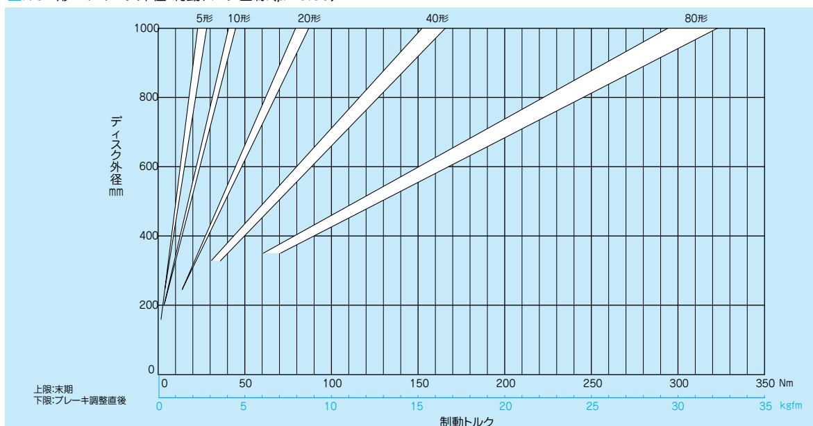
■NGB-5・10形
