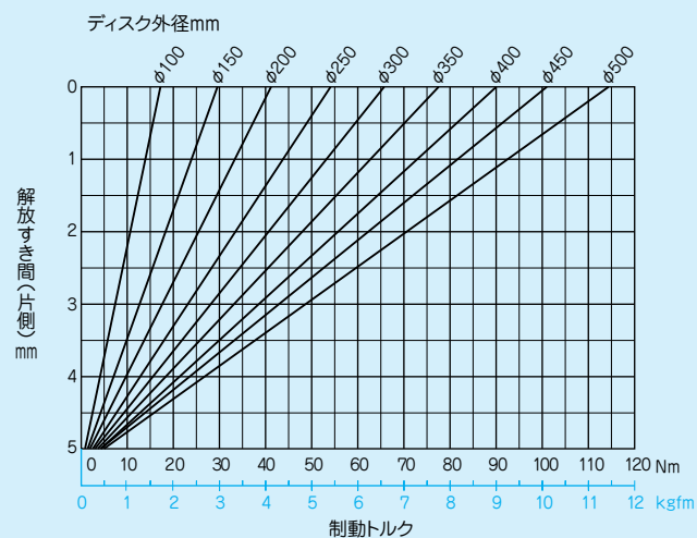
■NDB-20A形 初期解放すき間(片側)・制動トルク曲線( \mu=0.35 )
