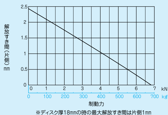
■NDB-1400A形 解放すき間(片側)・制動力曲線( \mu=0.33 )
