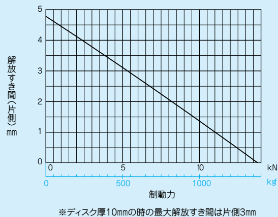
■NDB-1400B形 解放すき間(片側)・制動力曲線( \mu=0.33 )
