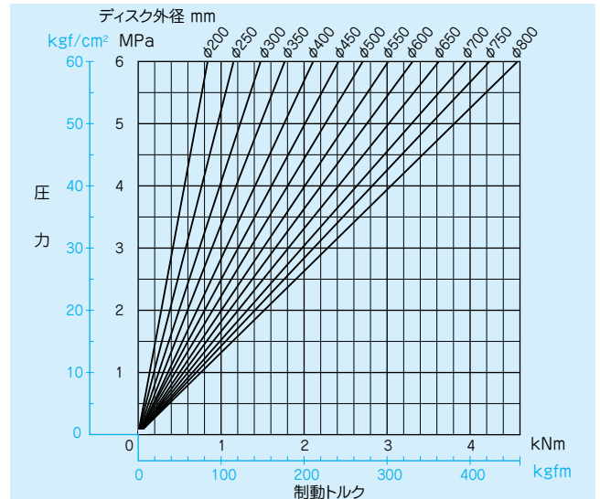
■ DBL-100 圧力・制動トルク曲線(μ=0.33)
