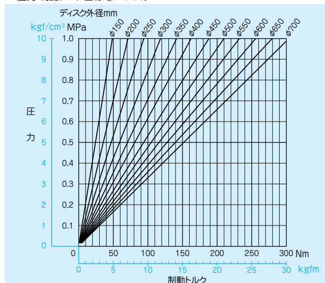
■DBA-20、DBL-20、RDB-20 圧力・制動トルク曲線 ( \mu=0.33 )
