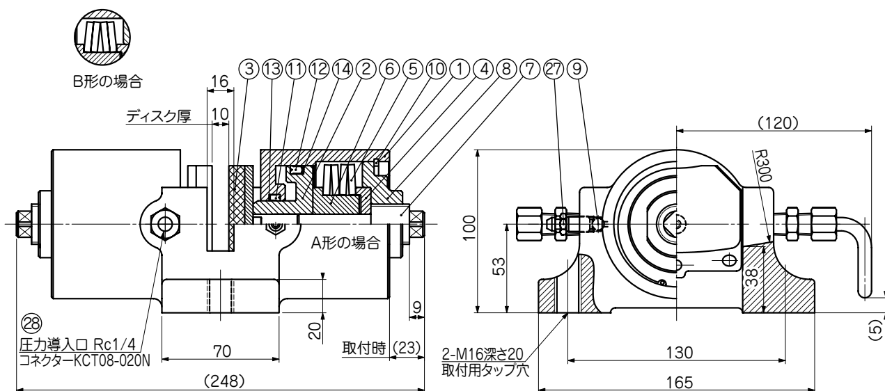
■NDB-1400形 部品表
