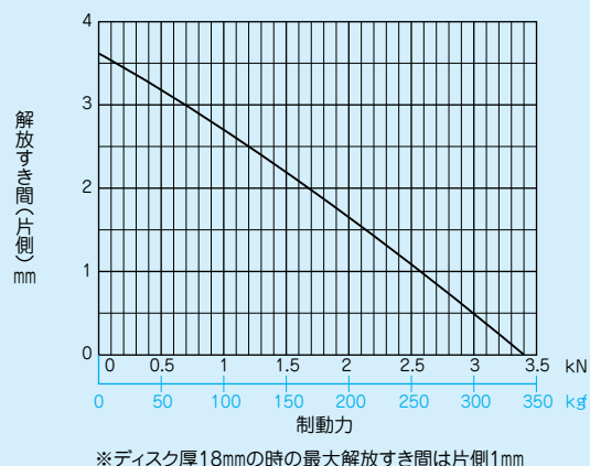
■NDB-400B形 解放すき間(片側)・制動力曲線( \mu=0.33 )
