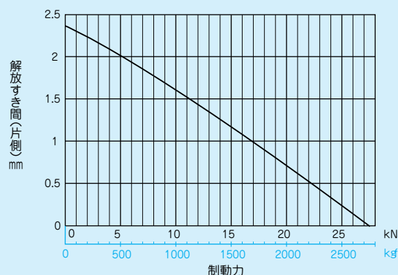
■NDB-1400B形 解放すき間(片側)・制動力曲線( \mu=0.33 )
