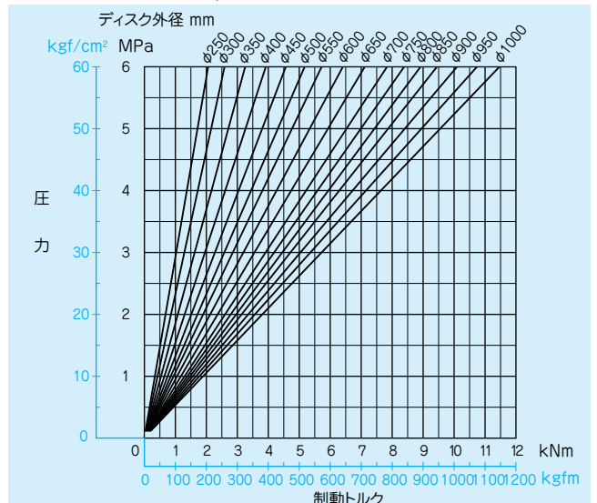
■ DBL-100 圧力・制動トルク曲線(μ=0.33)
