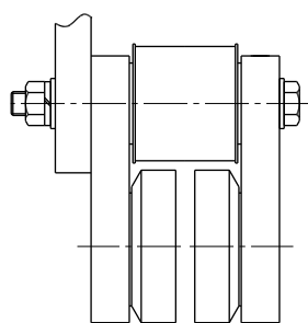
片側支持 (正常作動)
