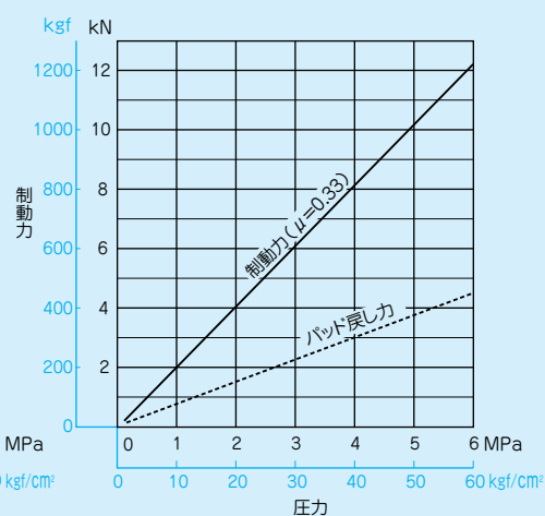
■RDB-50形
