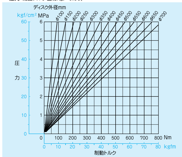
■DBL-20、RDB-20 圧力・制動トルク曲線 ( \mu=0.33 )
