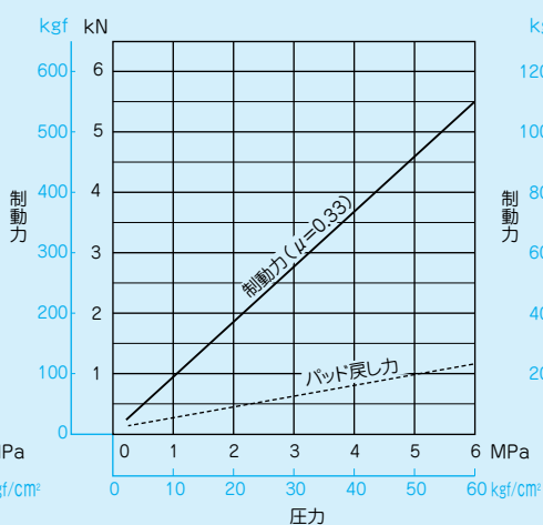
■RDB-20形
