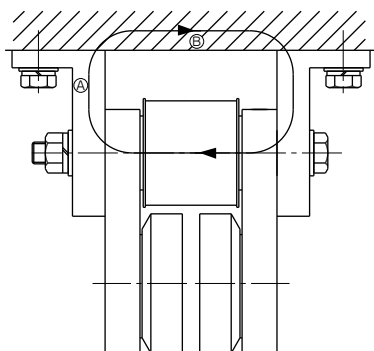
片側支持 (正常作動)
