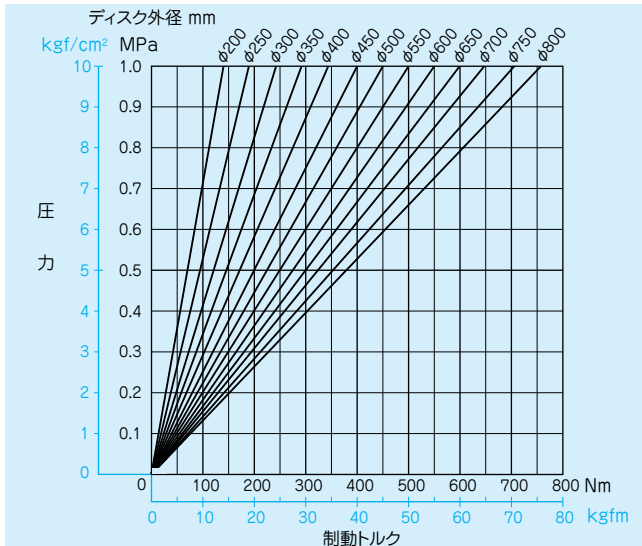
■ DBA-100、DBL-100 圧力・制動トルク曲線(μ=0.33)
