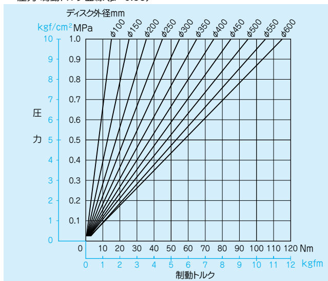
■DBA-20、DBL-20、RDB-20 圧力・制動トルク曲線 ( \mu=0.33 )
