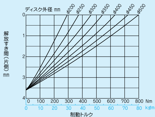
■NDB-400A形 解放すき間(片側)・制動トルク曲線( \mu=0.33 )
