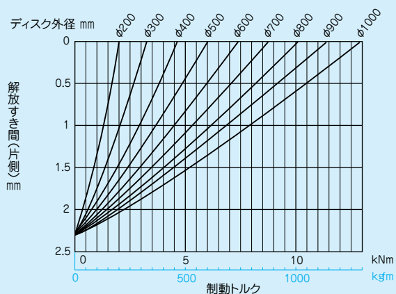
■NDB-1400B形 解放すき間(片側)・制動トルク曲線( \mu=0.33 )
